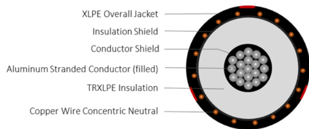
SERIES U35BTX
